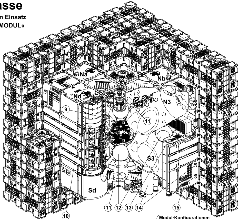
Modul-Konfigurationen
